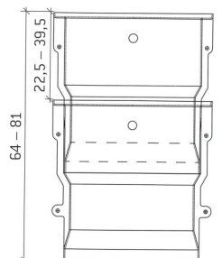
Placement de rehausse avec oeillets latéraux de fixation à couper (en cm)
