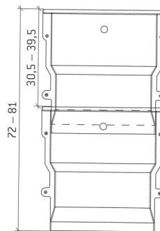
Placement de rehausse AVEC oeillets latéraux de fixation (en cm)
