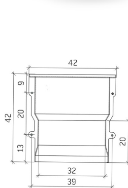
Dimensions courette d'aération (en cm)
