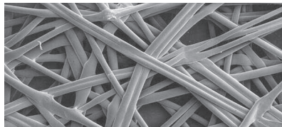
Plantex® Non Woven: gesündere Pflanzen, der Boden atmet, kein Ausfransen.
